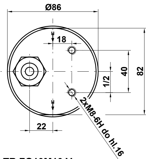
FILTR FG10M10 V s vizuální signalizací
